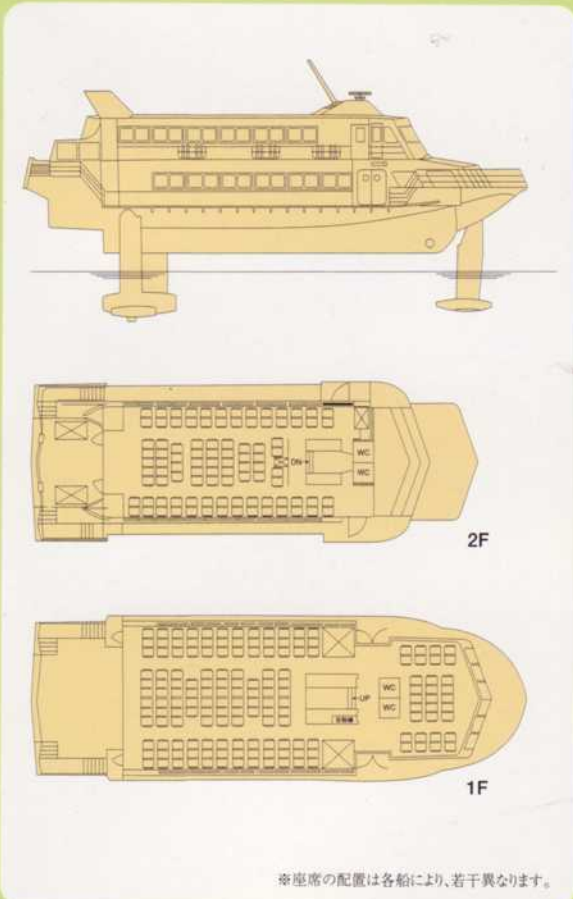
セブンアイランド 虹 ●総屯数/2811 ●深/2.59m ●全長(翼アップ)/30.78m ●最大速度/44.0kt ●全長(翼ダウン)/27.43m ●馬力/3800HP×2 ●巾/8.53m ●定員/260名
