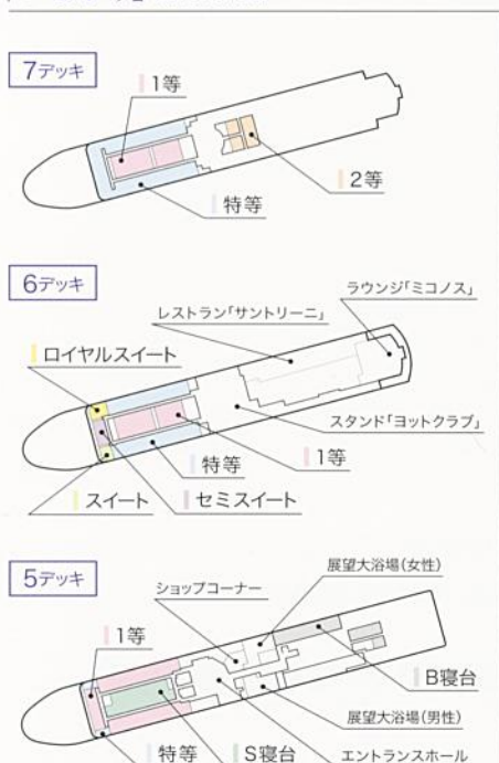
「いしかり」船内案内図
